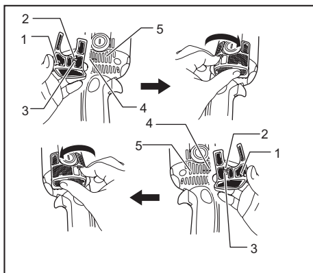
► 1. Crochet B 2. Crochet A 3. Nervure A 4. Évent A 5. Évent B
