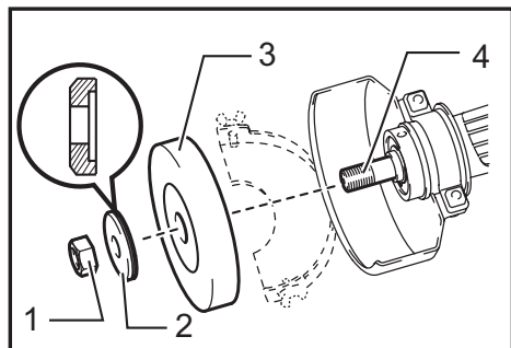
► 1. Écrou hexagonal 2. Flasque extérieur (type plat) 3. Meule 4. Axe
