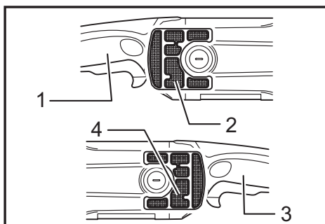
► 1. Poignée D 2. Accessoire pare-poussière D 3. Poignée G 4. Accessoire pare-poussière G
