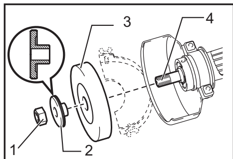
► 1. Écrou hexagonal 2. Flasque extérieur (type convexe) 3. Meule 4. Axe
