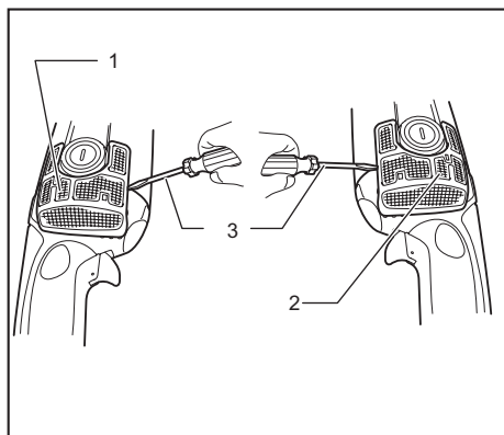
► 1. Accessoire pare-poussière D 2. Accessoire pare-poussière G 3. Tournevis
